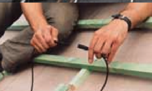
1. Montage randprofielen (IZEN). 2. Montage prefab panelen op draagstructuur (IZEN). 3. Afwerking dakbedekking (IZEN). 4. Opbouw dakgeïntegreerd systeem (Solar Technics). 5. Montage opbouw op leien dak (Lenoir Solar). 6. Onderlinge koppeling PV-panelen.
